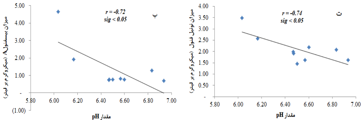
نمودار ۳- همبستگی بین مقادیر pH، COD و BOD با مقادیر بیسفنول A و نونیل فنول در نمونه‌های مورد مطالعه
