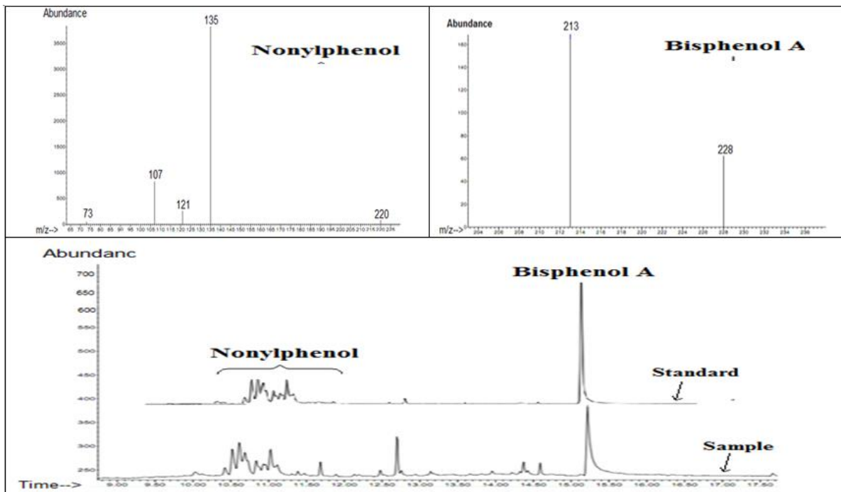
نمودار ۲- کروماتوگراف و یونهای انتخاب شده بیسفنول A و نونیل فنول در نمونه ها
