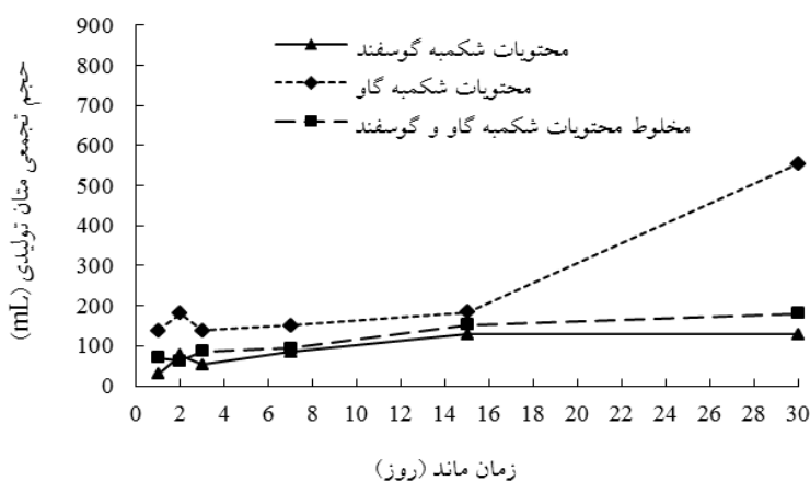
نمودار ۲- حجم تجمعی متان تولیدی در فرآیند هضم بی‌هوازی محتویات شکمبه
